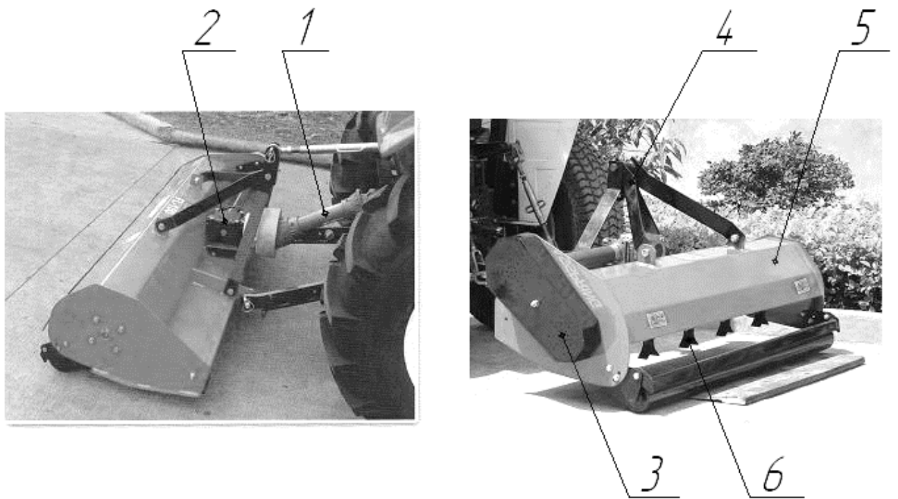
Рис.1 Устройство косилки
