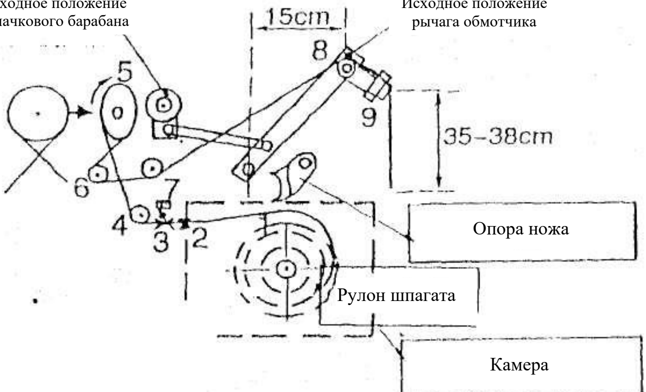
Рис. 4. Механизм обмотки
